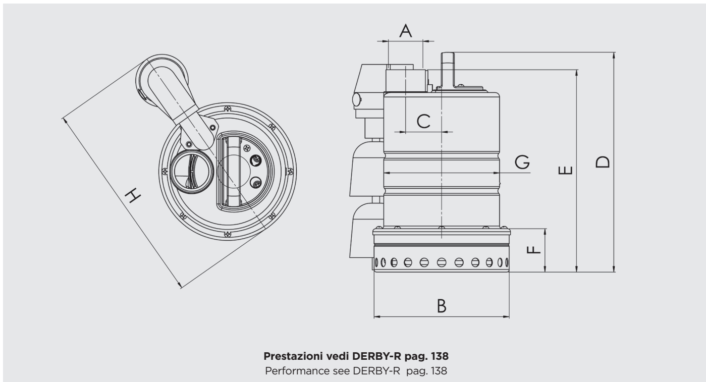
Elettropompe sommergibili con galleggiante verticale Submersible electric pumps with vertical float
